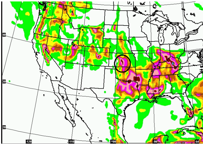
Figur 4. RUC (Rapid Update Cycle) og NAM (North American Mesoscale) modelresultater, der viser 0-3 km CAPE værdier. Begge modeller kommer fra NOAA's NCEP (National Center for Environmental Prediction). De to første figurer viser 12 timers prognoser frem til 5. maj kl. 0 UTC fra hhv. RUC og NAM; den sidste figur viser en 18 timers prognose frem til 5. maj kl. 6 UTC fra NAM. Cirklene viser at der er høje værdier det samme sted som SRH-CAPE kombinationen viste høje værdier (figur 3).
