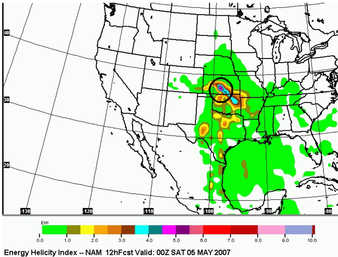
Figur 3. Energy Helicity Index (EHI) fra en NAM (North American Mesoscale) modelkørsel, der viser et område, markeret med cirkel, med forudsagt forhøjet SRH og CAPE i det centrale og sydlige Kansas.
