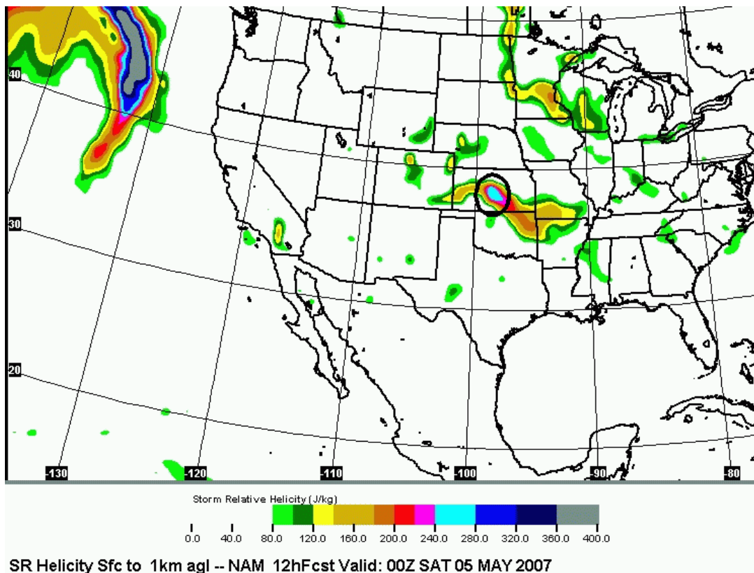
Figur 2. Storm Relative Helicity (SRH) fra en NAM (North American Mesoscale) modelkørsel i den første kilometer af atmosfæren, viste et forudsagt maksimum tæt på en varmfront i det centrale Kansas. (se cirkel). SRH kan betragtes som et mål for mulig tornadoaktivitet.
